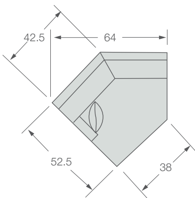
2145-WL Ethan Left Arm Wedge W75 D52.5 H34
